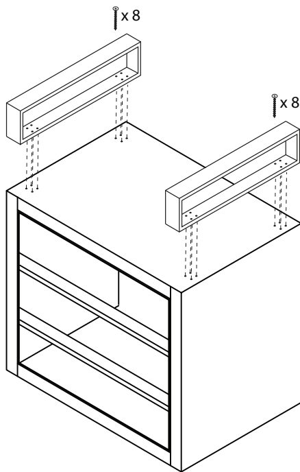
S-FEET
